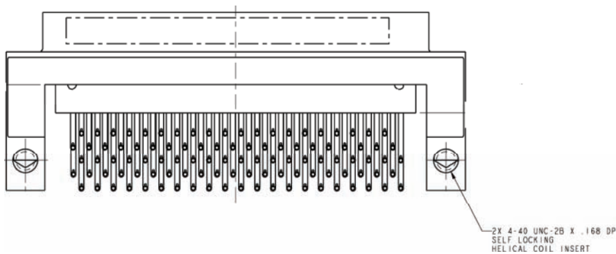
Receptacle - Socket
